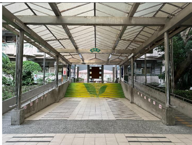
當年未考量相關規定或沒有相關規定，或受限空間因素，坡道過於陡直，經測量約為 1:8.6
